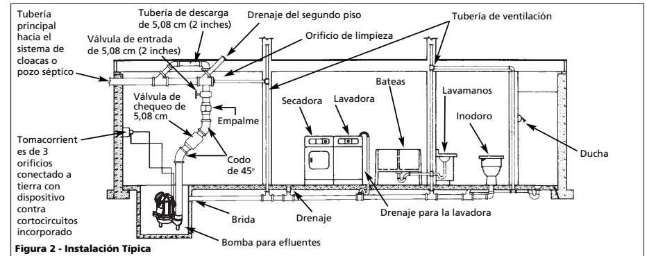
Figura 2 - Instalación Típica
