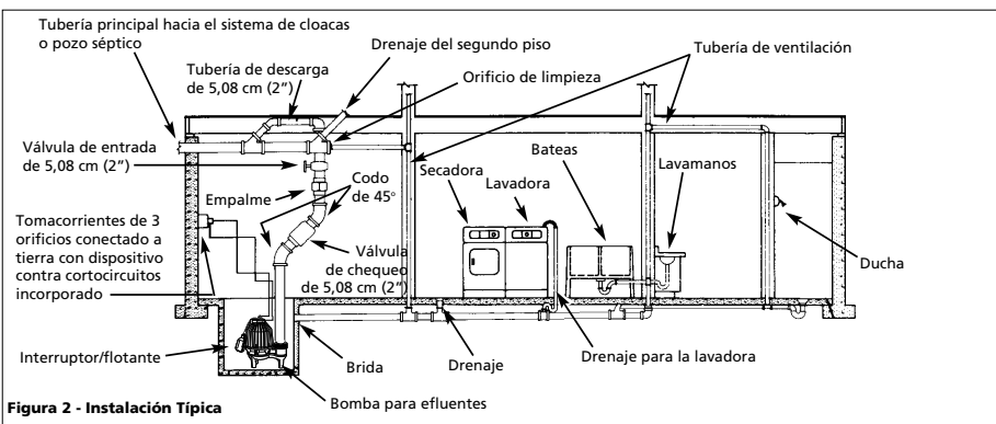
Figura 2 - Instalación Típica
