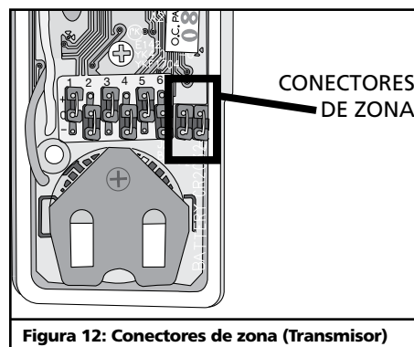
Figura 12: Conectores de zona (Transmisor)
