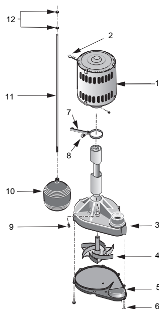
Modèle 5020B-04
