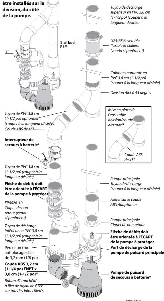
Fig 3 : Installation typique avec tuyau de décharge commun.
