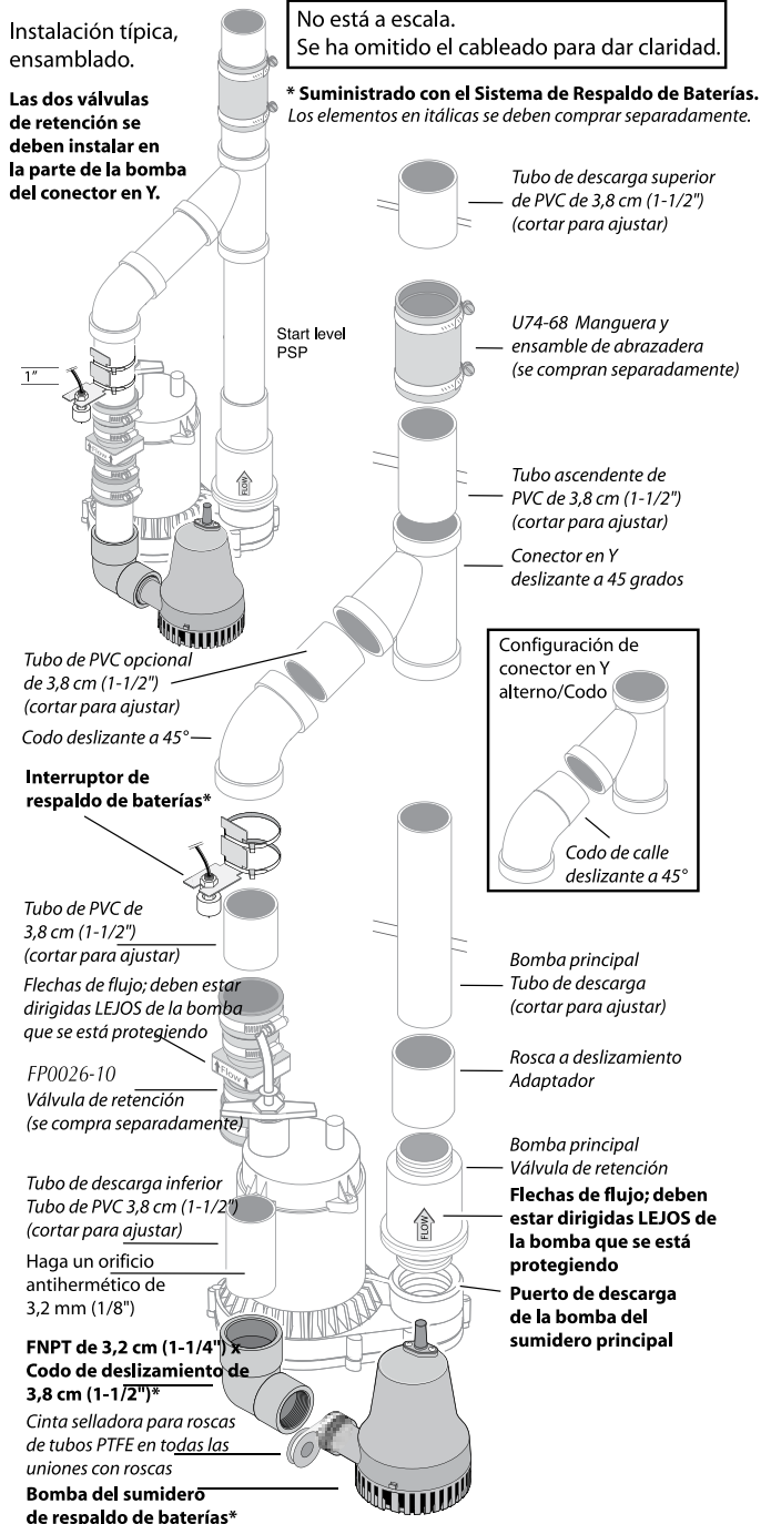
Figura 3: Instalación típica con tubos de descarga comunes.
